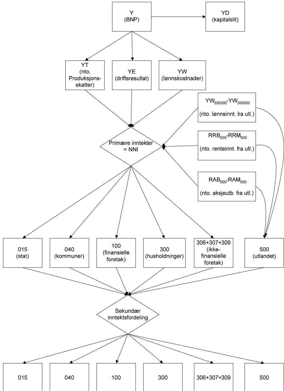
Figur 8.2.1. Strukturen i inntektsregnskapet i MODAG (modellens variabelsymbol i kursiv)
