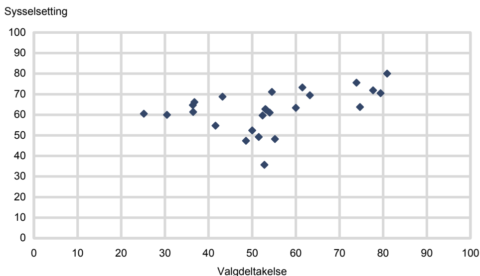
Figur 5.1. Andelen som er sysselsatt blant alle bosatte 4. kvartal 2008, og andel stemmeberettigede som deltok ved stortingsvalget 2009 for 25 land 1
