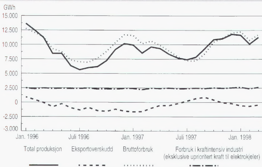
Produksjon, forbruk og eksportoverskudd av elektrisk kraft per måned. Januar 1996-mars 1998. GWh
