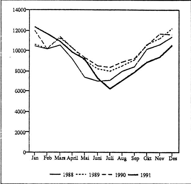
Figur 2. Produksjon av elektrisk kraft. Måned. GWh
