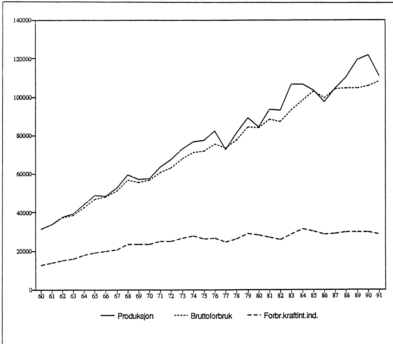
Figur 6. Produksjon, bruttoforbruk og forbruk i kraftintensiv industri. 1960 - 1991. GWh
