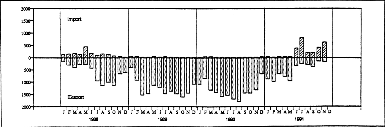
Figur 4. Import og eksport av elektrisk kraft. Måned. GWh
