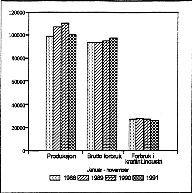
Figur 2. Produksjon, brutto forbruk og forbruk i kraftintensiv industri. Januar-november. GWh
