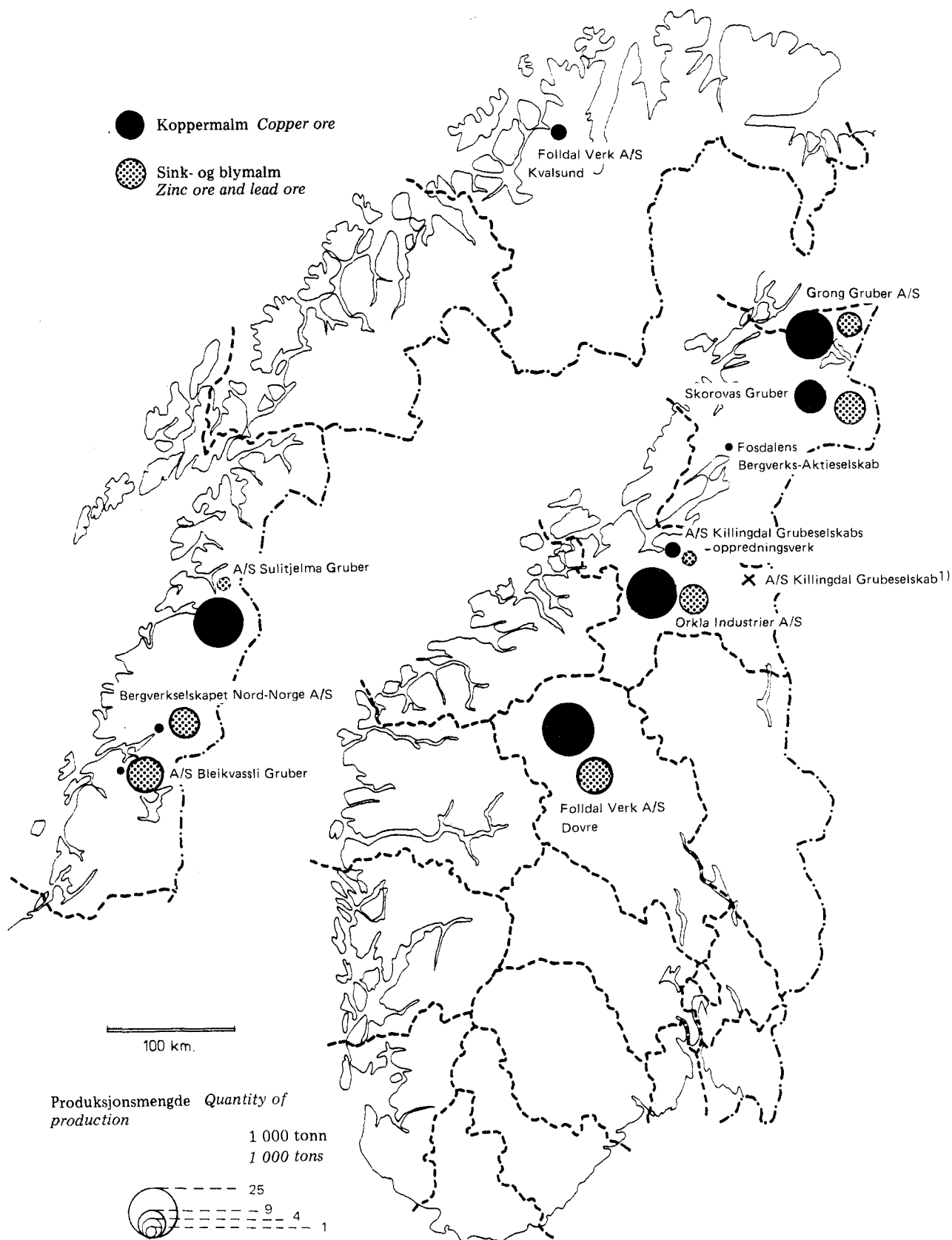
Figur 12. Produksjonsmengde og beliggenhet. Koppermalm-, sink- og blymalmgruver. Se tabell 58, side 200 Quantity of production and location. Mines of copper ore, zinc ore and lead ore. See table 58, page 200
