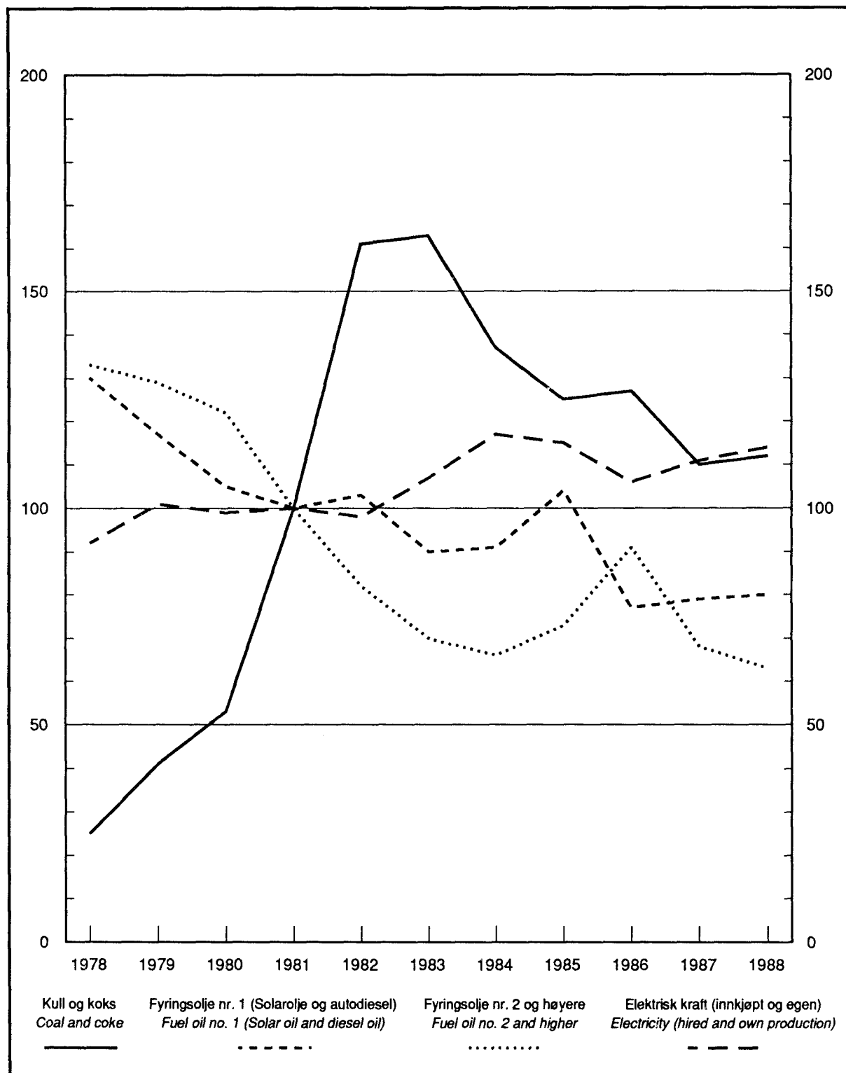
Figur 1. Forbruk av brensel og elektrisk kraft i store bedrifter. 1978-1988. Relative tall. 1981=100 (beregnet ut fra mengdeoppgavene) 1) Consumption of fuel and electric energy in large establishments. 1978-1988. Proportionate figures. 1981=100 (calculated on data of quantity) 1)
