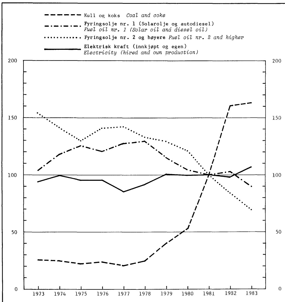
Figur 1. Forbruk av brensel og elektrisk kraft i store bedrifter. 1973-1983. Relative tall. 1981 = 100 (beregnet ut fra mengdeoppgavene) 1) Consumption of fuel and electric energy in large establishments. 1973-1983. Proportionate figures. 1981=100 (calculated on data of quantity)
