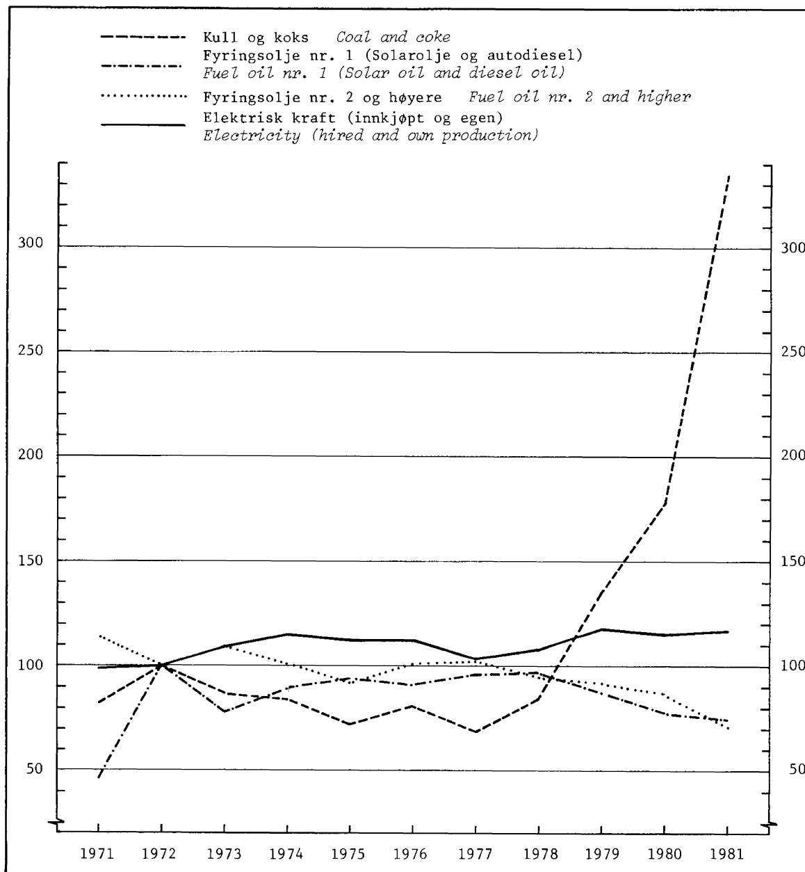
Figur 3. Forbruk av brensel og elektrisk kraft i store bedrifter, 1971-1981. Relative tall. 1972 = 100 (beregnet ut fra mengdeoppgavene) 1) Consumption of fuel and electric energy in large establishments. 1971-1981. Proportionate figures. 1972=100 (calculated on data of quantity)
