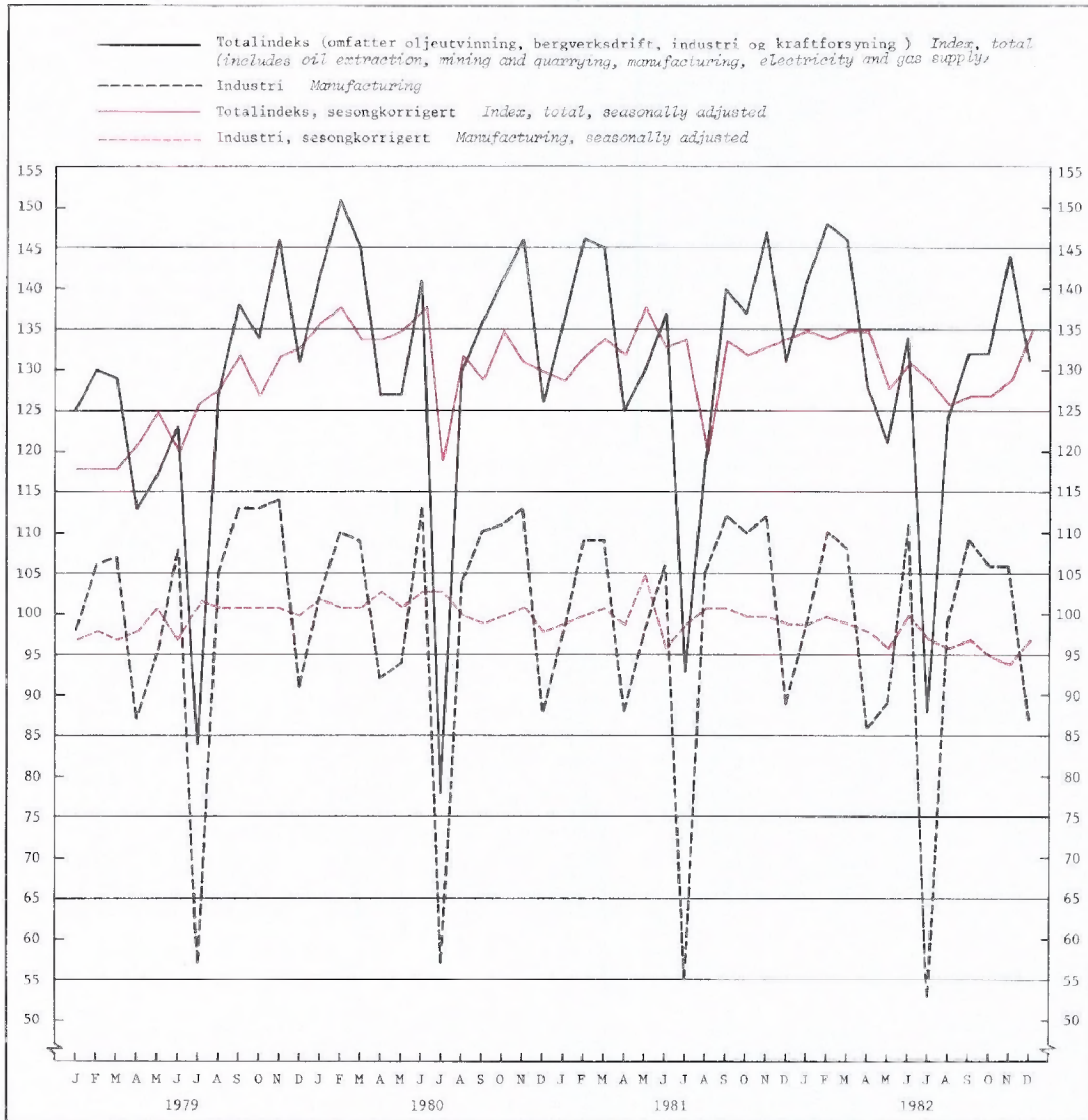
Figur 2. Produksjonsindeks (bruttoprodukt). Månedlig, 1975 = 100 Index of industrial production (value added). Monthly. 1975 = 100
