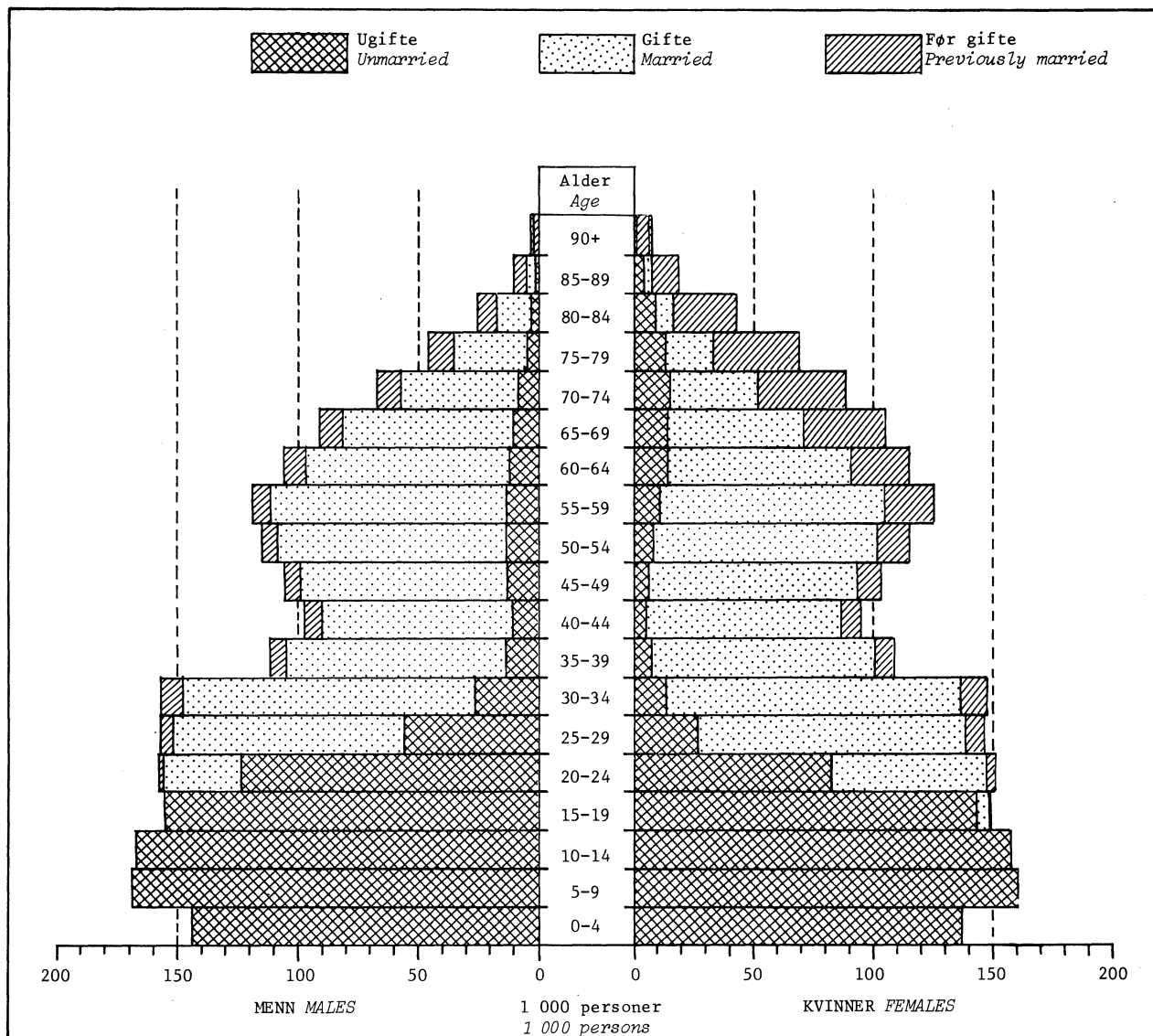
Figur 1. Folkemengden etter kjønn, alder og ekteskapelig status, se tabell 3 Population by sex, age and marital status, see table 3
