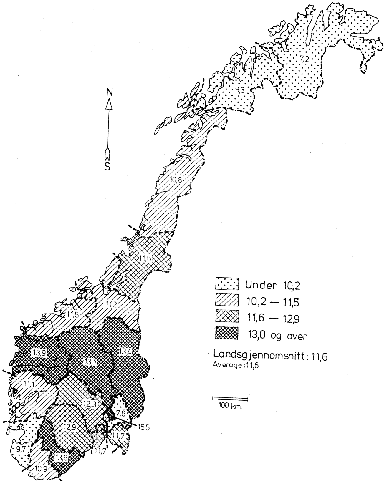
Figur 3. Personer 67 år og over i prosent av folkemengden i alt. Fylker. Landsgjennomsnitt: 11,6 Persons of age 67 years and over as percentage of total population. Counties. Average: 11.6
