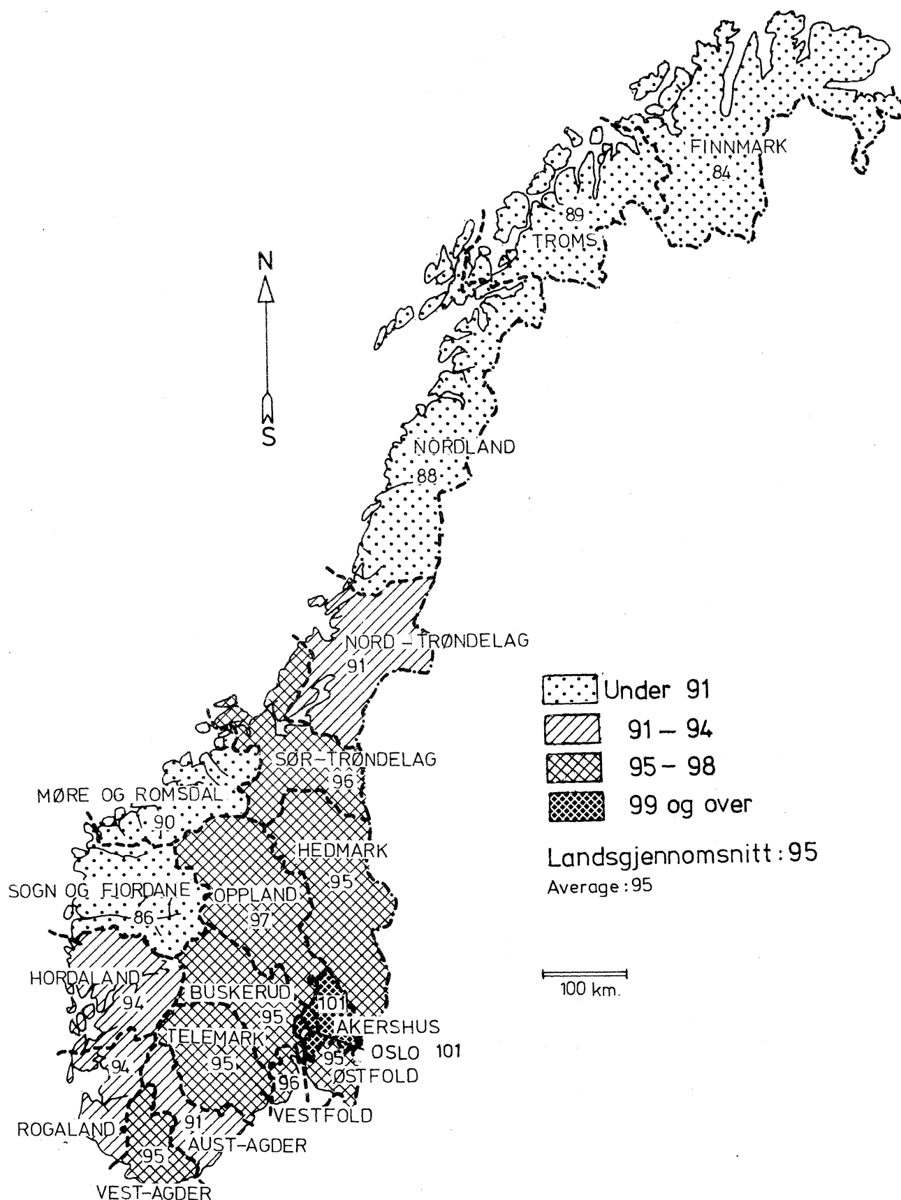
Figur 2. Kvinner pr. 100 menn i aldersgruppen 20-39 år. Fylker. Lands- gjennomsnitt: 95 Females per 100 males in age group 20-39 years. Counties. Average: 95
