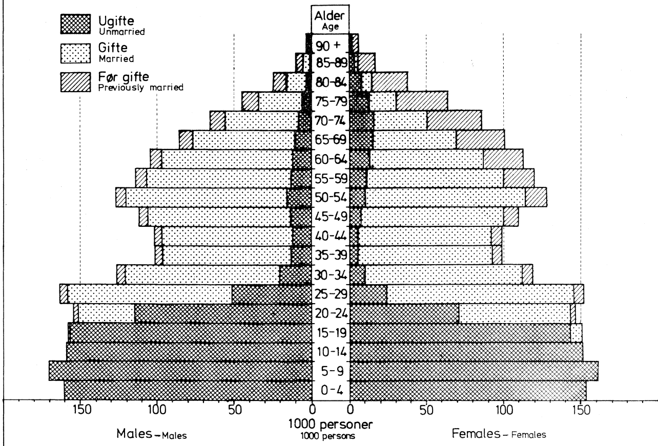
FIGUR 1. FOLKEMENGDEN ETTER KJØNN, ALDER OG EKTESKAPELIG STATUS, SE TABELL 3. POPULATION BY SEX, AGE AND MARITAL STATUS, SEE TABLE 3.
